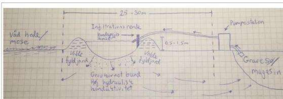
Figur 3: Principkitse for infiltrationssøen. Vandets bevægelser er indikeret med pile.
