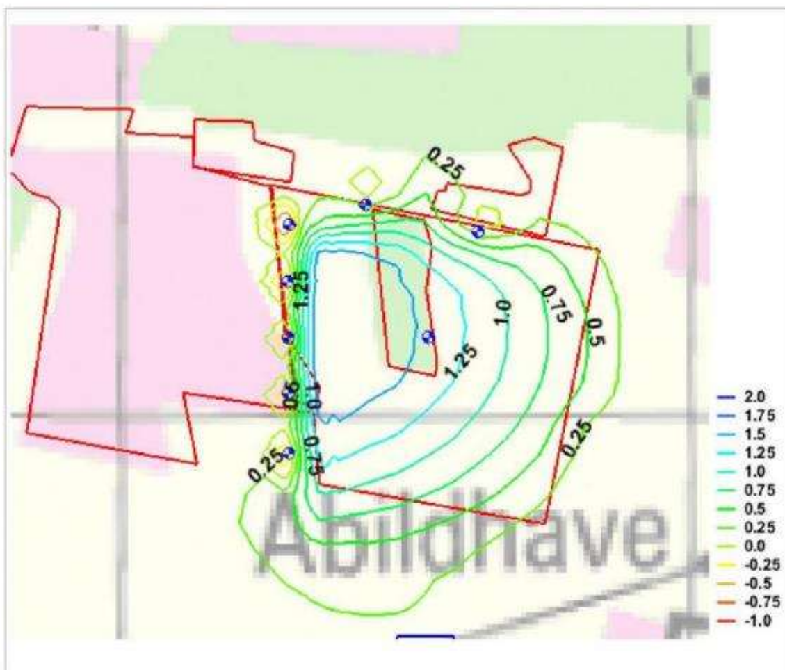
Figur 5: Maksimalde sænkninger der kan forventes i grundvandspejl under gravearbejdet illustreret med 0.25m isolinjer.
