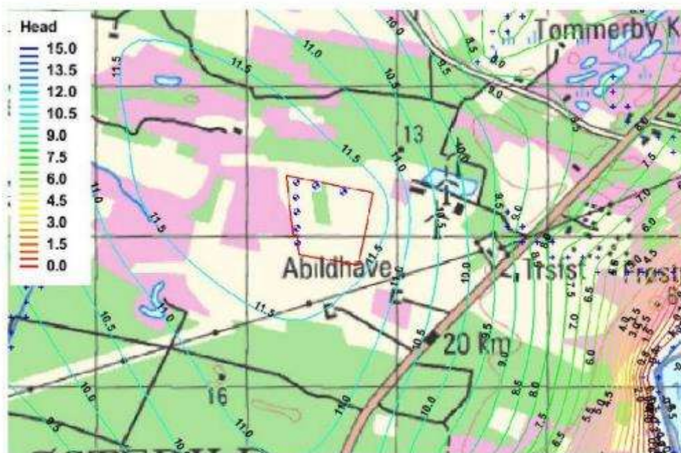
Figur 2-8 Scenarie 2- Vandspejlskoter (m) efter etablering af gravesø med infiltrationsrende (15 m 3 /t)
