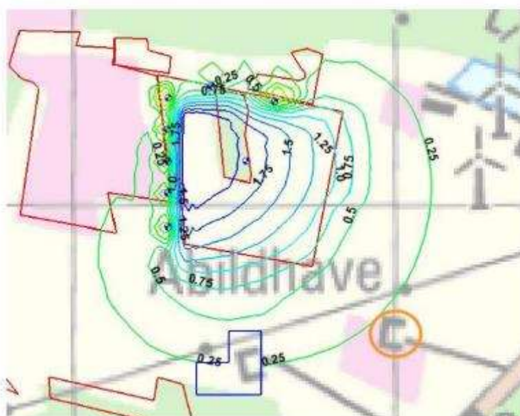
Figur 3-8 Scenarie 6 - Sænkning i modellag 1
