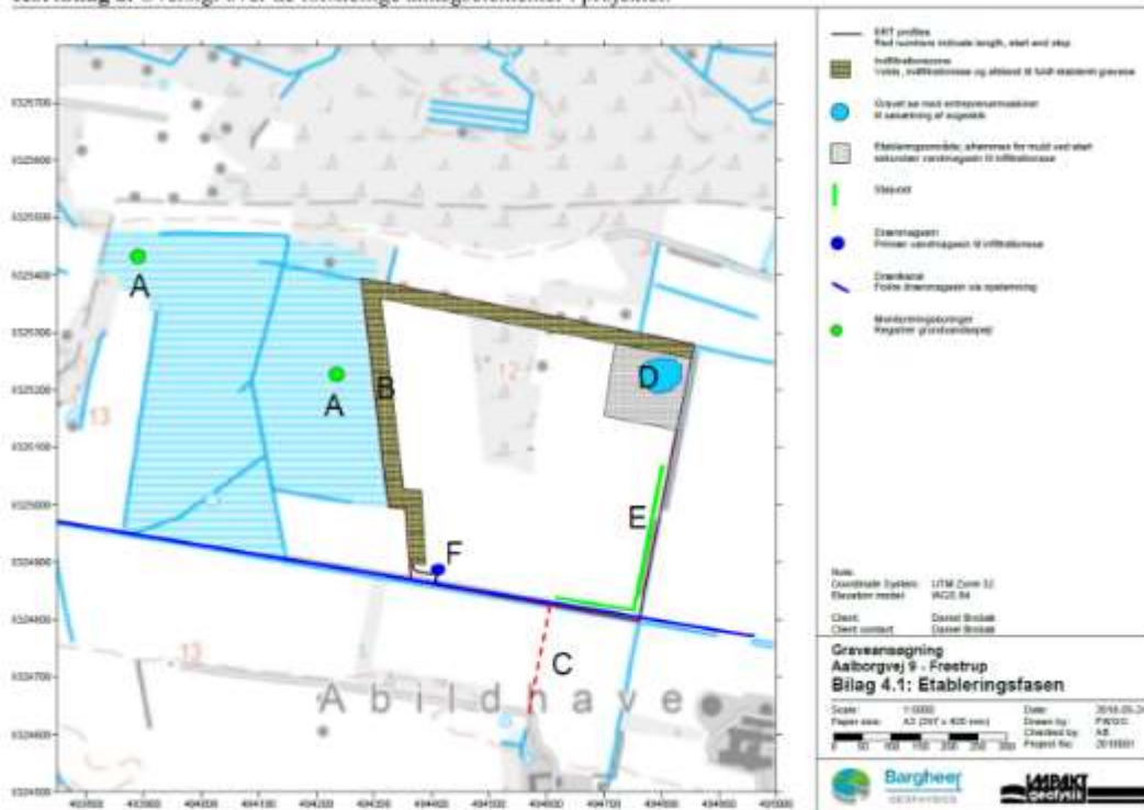
Kortbilag 2. Oversigt over de forskellige anlægselementer i projektet.
