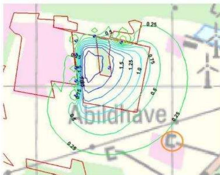
Figur 3-9 Scenario 6 – Sænkning i modellag 2
